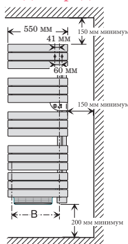
Вид спереди
